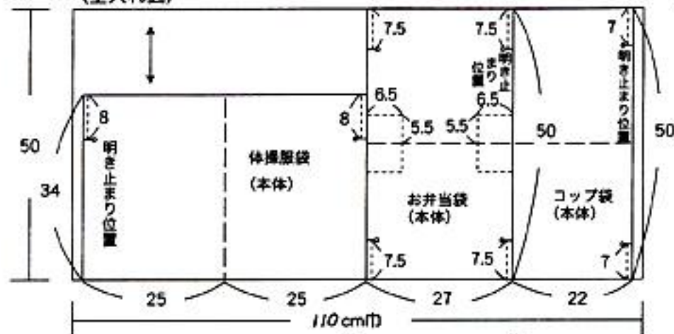
〈型入れ図〉
